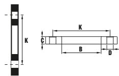
Brida plana acero zincado para portabrida PVC Zinc plated steel plain flange for PVC adaptor Bride plate de sûreté en acier zingué pour collet PVC
