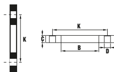
Brida plana acero zincado para portabrida PE Zinc plated steel security plain flange for PE adaptor Bride plate de sûreté en acier zingué pour porte bride PE
