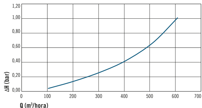
Válvulas / Valves DN 250
