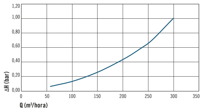
Válvulas / Valves DN 150
