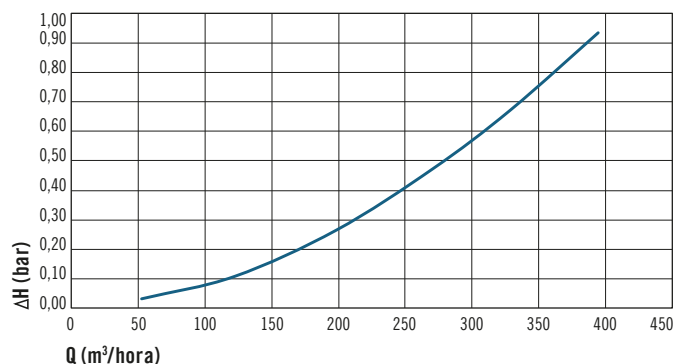
Válvulas / Valves DN 200
