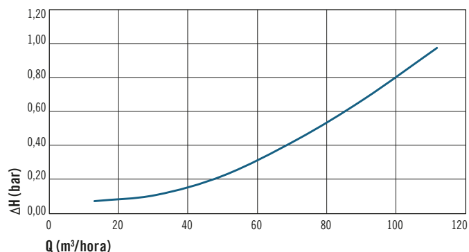
Válvulas / Valves DN 100
