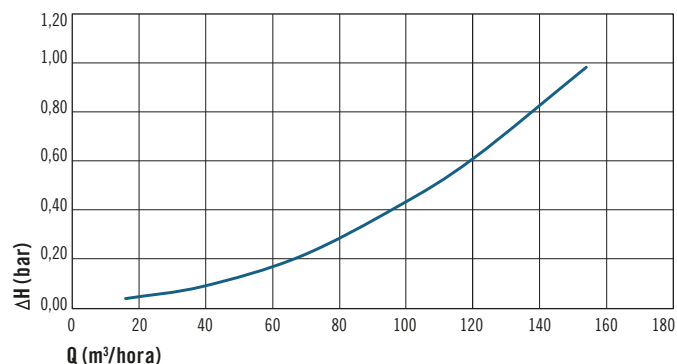
Válvulas / Valves DN 110
