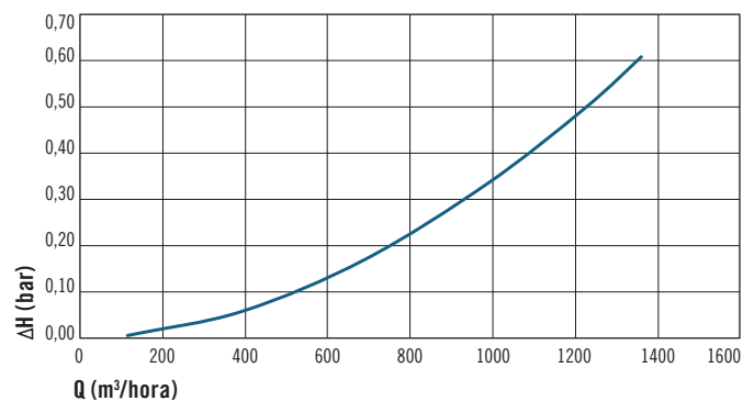
Válvulas / Valves DN 250
